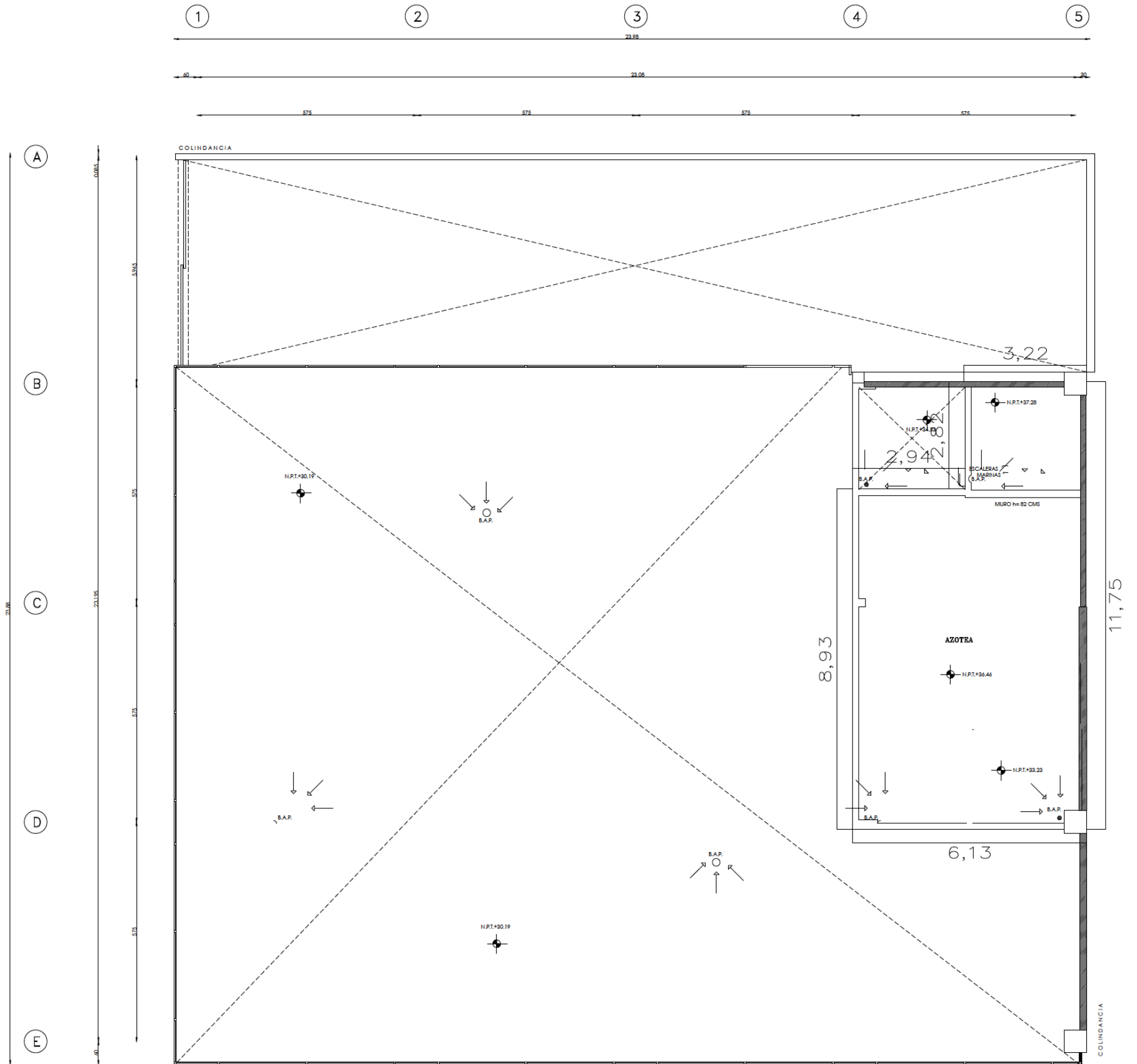
PLANTA AZOTEA
